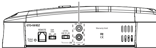
Connecteurs d'entrée
